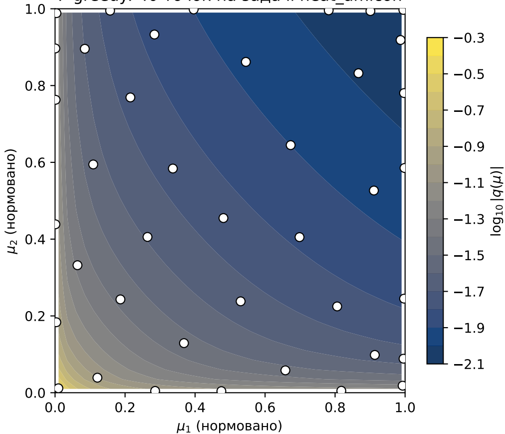
P-greedy: 40 точок на задачі heat_amicon
